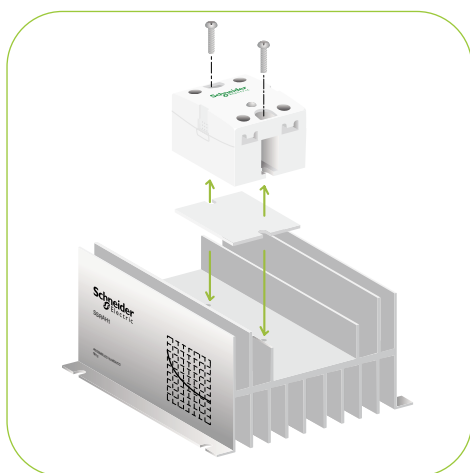
SSRP通过底板安装在散热槽上
